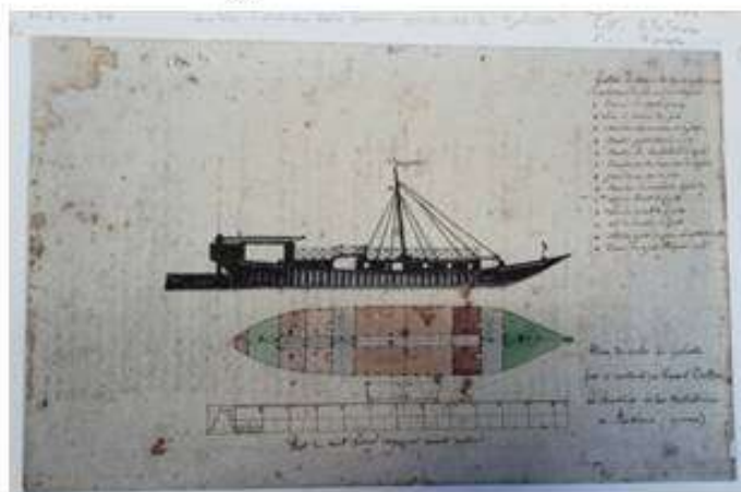
Plan original d'une Galiote en 1800
