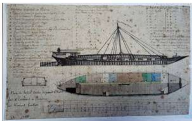
Plan original du Saint Victor en 1800
